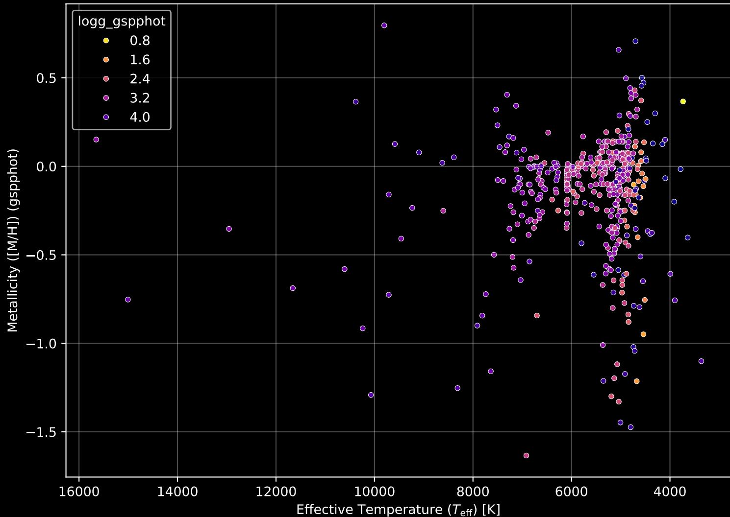
APOGEE DR17 Field: [150+04] Stellar Population Parameters (n= 459)
